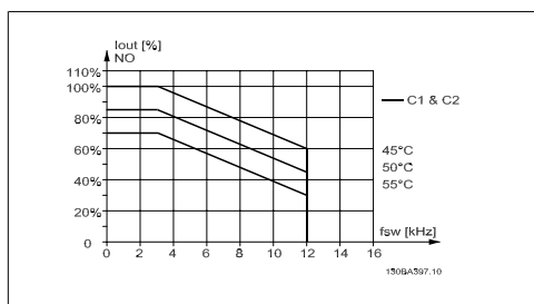
Ilustracja 4.11: Obniżanie wartości znamionowych I_{out} dla różnych T_{AMB, MAX} dla obudowy C za pomocą 60 PWM w trybie zwykłego momentu obrotowego (obrót maks. 110%)
