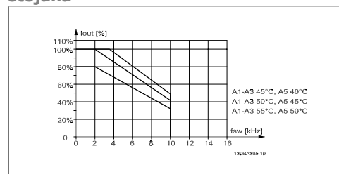
Ilustracja 4.2: Obniżanie wartości znamionowych I_{out} dla różnych T_{AMB, MAX} dla obudowy A za pomocą SFAVM
