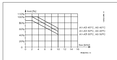
Ilustracja 4.4: Obniżanie wartości znamionowych I_{out} dla różnych T_{AMB, MAX} dla obudowy A za pomocą SFAVM i kabla silnikowego o maks. długości 10 m
