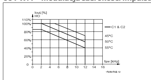
Ilustracja 4.9: Obniżanie wartości znamionowych I_{out} dla różnych T_{AMB, MAX} dla obudowy C za pomocą 60 PWM w trybie wysokiego momentu obrotowego (obrót maks. 160%)
