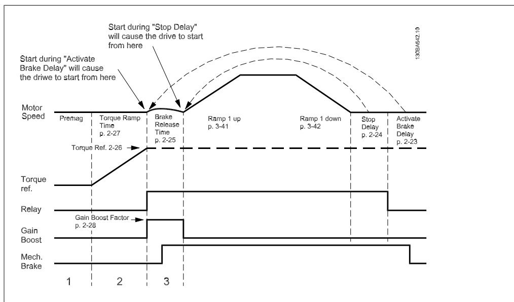
Ilustracja 3.4: Sekwencja zwolnienia hamulca dla sterowania hamulca mechanicznego
