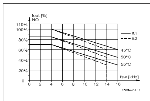
Ilustracja 4.7: Obniżanie wartości znamionowych I_{out} dla różnych T_{AMB, MAX} dla obudowy B za pomocą 60 PWM w trybie zwykłego momentu obrotowego (obrót maks. 110%)
