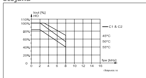
Ilustracja 4.10: Obniżanie wartości znamionowych I_{out} dla różnych T_{AMB, MAX} dla obudowy C za pomocą SFAVM w trybie wysokiego momentu obrotowego (obrót maks. 160%)
