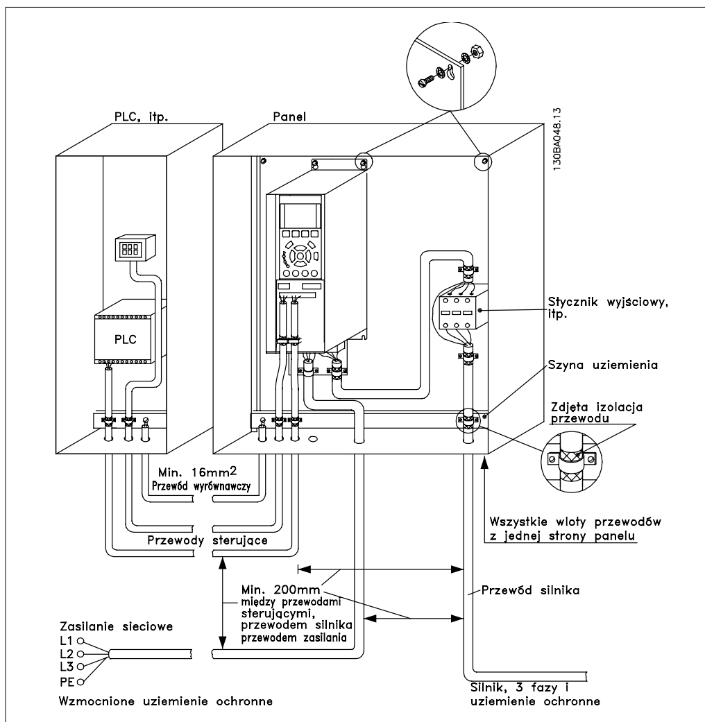
Ilustracja 6.14: Podłączenie złączy elektrycznych przetwornicy częstotliwości w szafie zgodnie z EMC.
