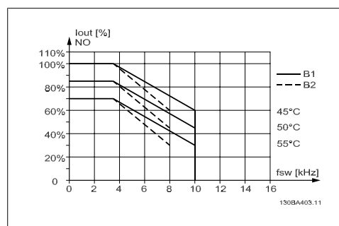
Ilustracja 4.8: Obniżanie wartości znamionowych I_{out} dla różnych T_{AMB, MAX} dla obudowy B za pomocą SFAVM w trybie zwykłego momentu obrotowego (obrót maks. 110%)
