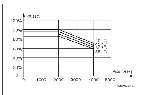
Ilustracja 4.20: Obniżanie wartości znamionowych I_{out} dla różnych T_{AMB, MAX} dla obudowy D przy 690 V za pomocą SFAVM w trybie zwykłego momentu obrotowego (obrót maks. 110%) Uwaga: nie dotyczy P315.
