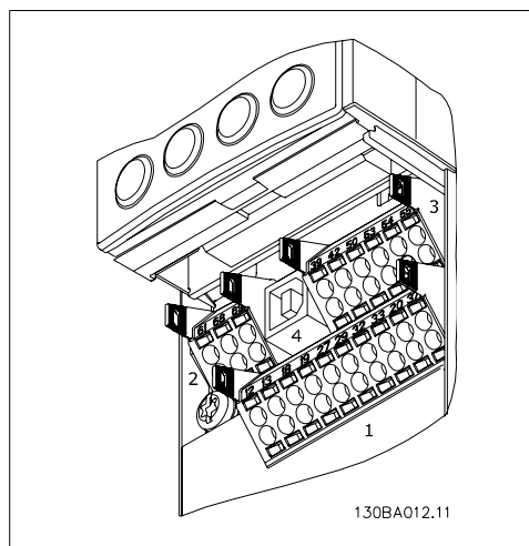
Ilustracja 6.11: Zaciski sterowania (wszystkie obudowy)
