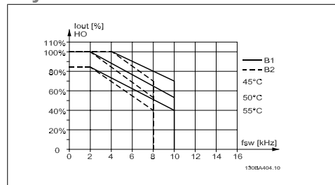
Ilustracja 4.6: Obniżanie wartości znamionowych I_{out} dla różnych T_{AMB, MAX} dla obudowy B za pomocą SFAVM w trybie wysokiego momentu obrotowego (obrót maks. 160%)
